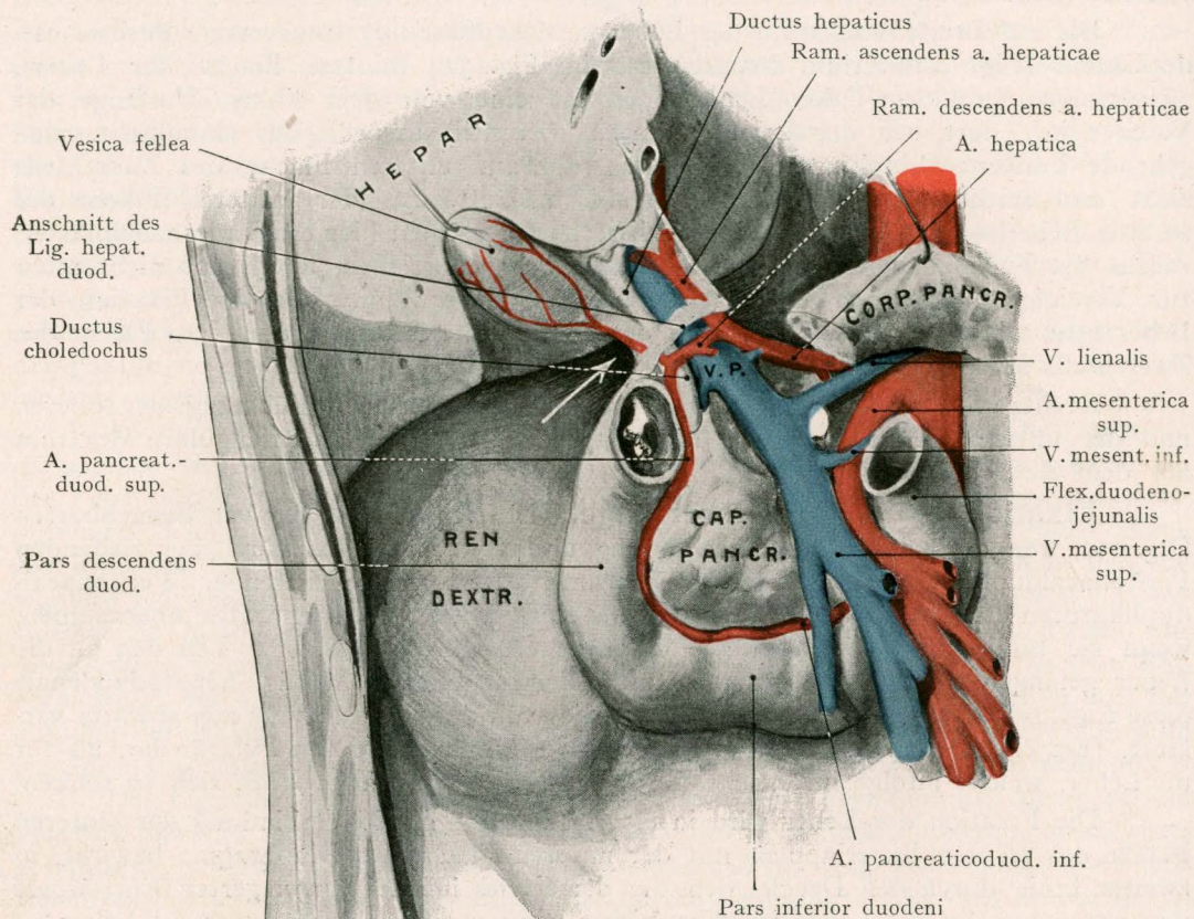
Fig. 327. Topographie des Lig. hepatoduodenale und der V. portae. Ein Teil des Pankreaskörpers ist abgetragen worden. Der Pfeil gibt das Foramen epiploicum an. V. P. V. portae.
